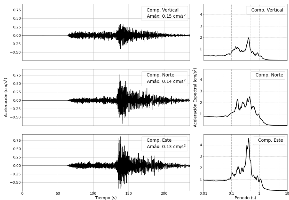
Figura 7: Registros de aceleracion para el sismo del 25/05/2026 (M6.5) y sus correspondientes espectros de respuestas con amortiguamiento al 5 %
