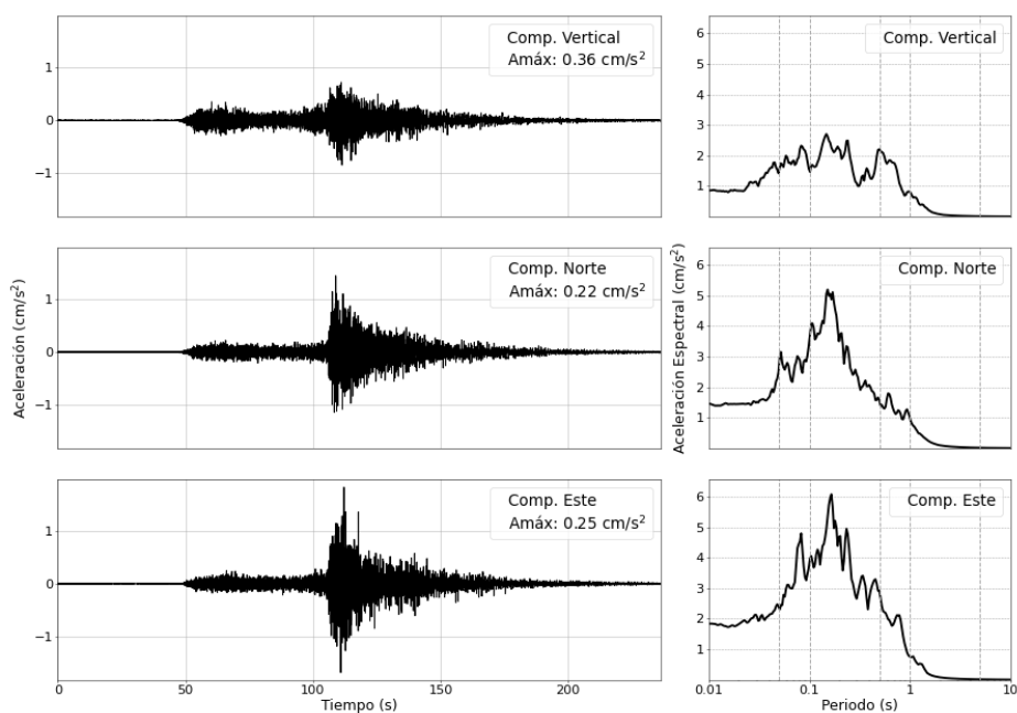
Figura 5: Registros de aceleracion para el sismo del 25/05/2026 (M6.5) y sus correspondientes espectros de respuestas con amortiguamiento al 5 %
