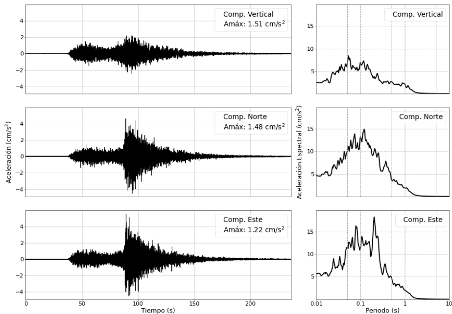
Figura 3: Registros de aceleración para el sismo del 25/05/2026 (M6.5) y sus correspondientes espectros de respuestas con amortiguamiento al 5 %
