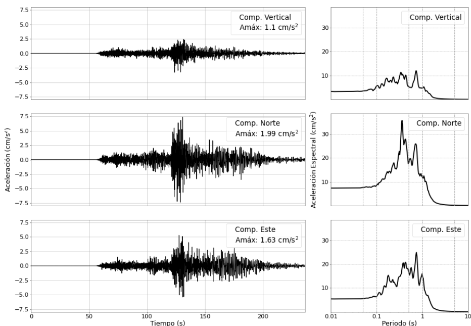
Figura 6: Registros de aceleración para el sismo del 25/05/2026 ( M_{6.5} ) y sus correspondientes espectros de respuestas con amortiguamiento al 5 %
