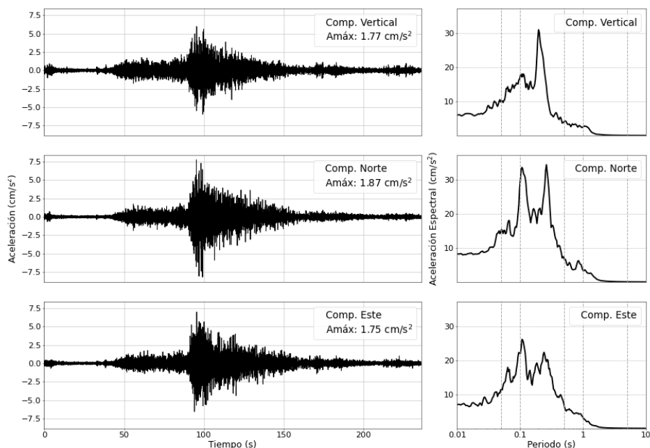
Figura 4: Registros de aceleracion para el sismo del 25/05/2026 (M6.5) y sus correspondientes espectros de respuestas con amortiguamiento al 5 %
