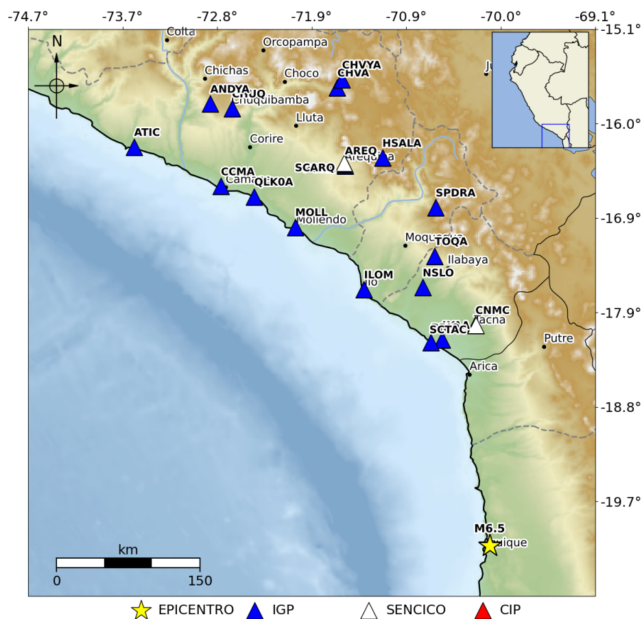
Figura 1: Epicentro del sismo ocurrido el 25/05/2026 y distribución de las estaciones acelerométricas consideradas en este reporte
