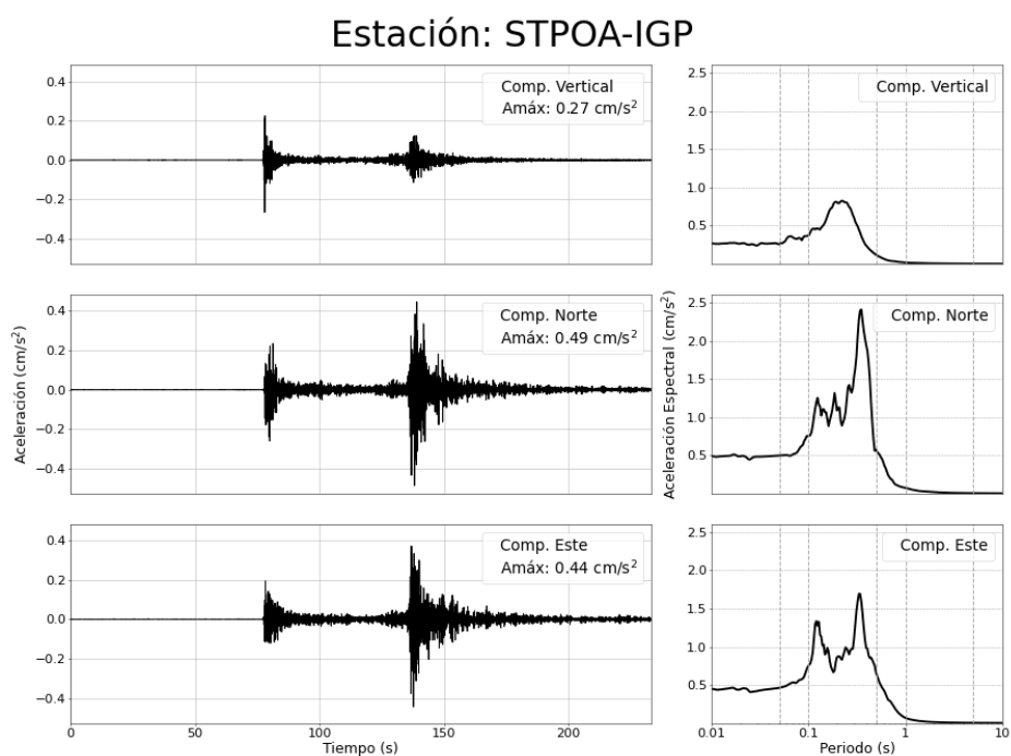
Figura 4: Registro de aceleración para el sismo del 03/08/2025 (M5.5) y sus correspondientes espectros de respuestas con amortiguamiento al 5 %
