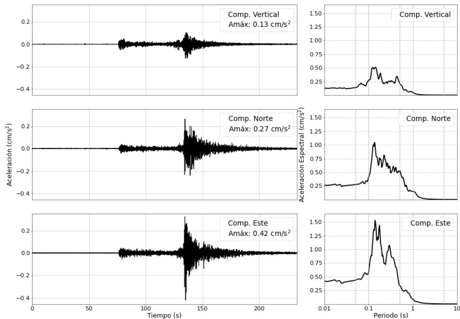
Figura 3: Registros de aceleración para el sismo del 03/08/2025 (M5.5) y sus correspondientes espectros de respuestas con amortiguamiento al 5 %
