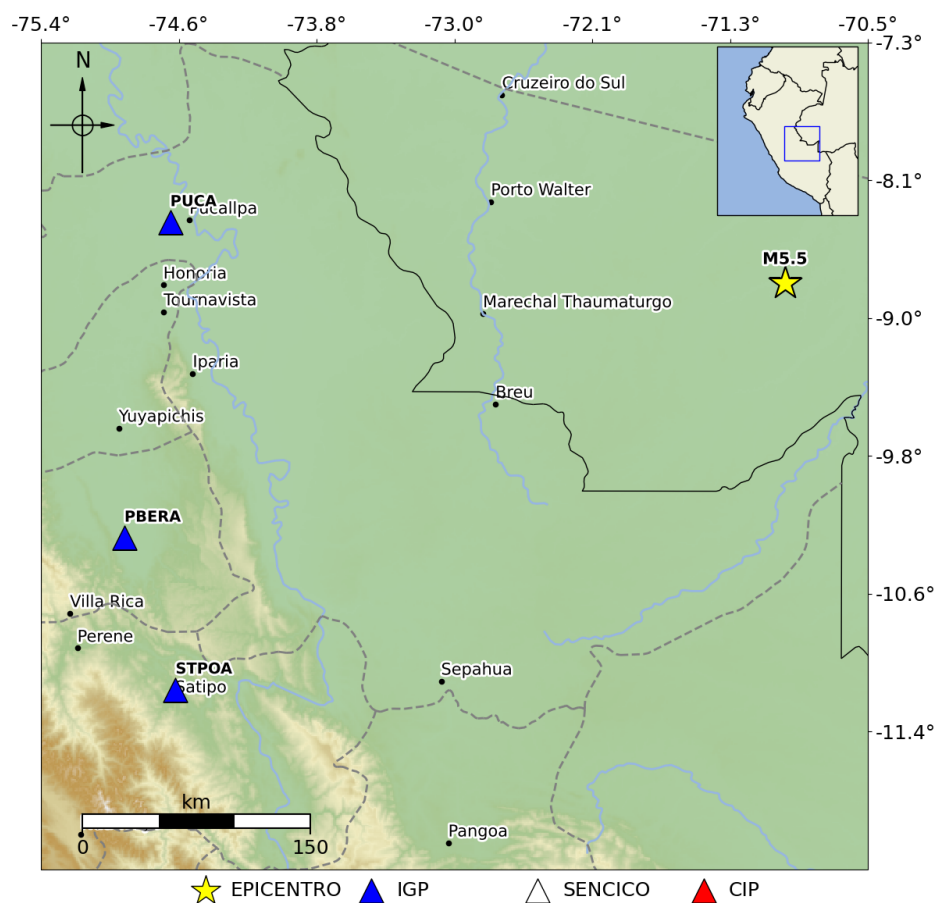
Figura 1: Epicentro del sismo ocurrido el 03/08/2025 y distribución de las estaciones acelerométricas consideradas en este reporte
