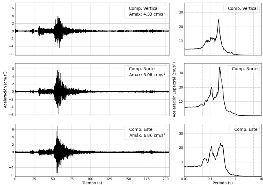
Figura 3: Registros de aceleración para el sismo del 23/08/2025 (M5.2) y sus correspondientes espectros de respuestas con amortiguamiento al 5 %
