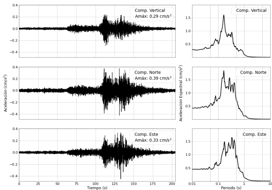
Figura 6: Registros de aceleración para el sismo del 23/08/2025 (M5.2) y sus correspondientes espectros de respuestas con amortiguamiento al 5 %
