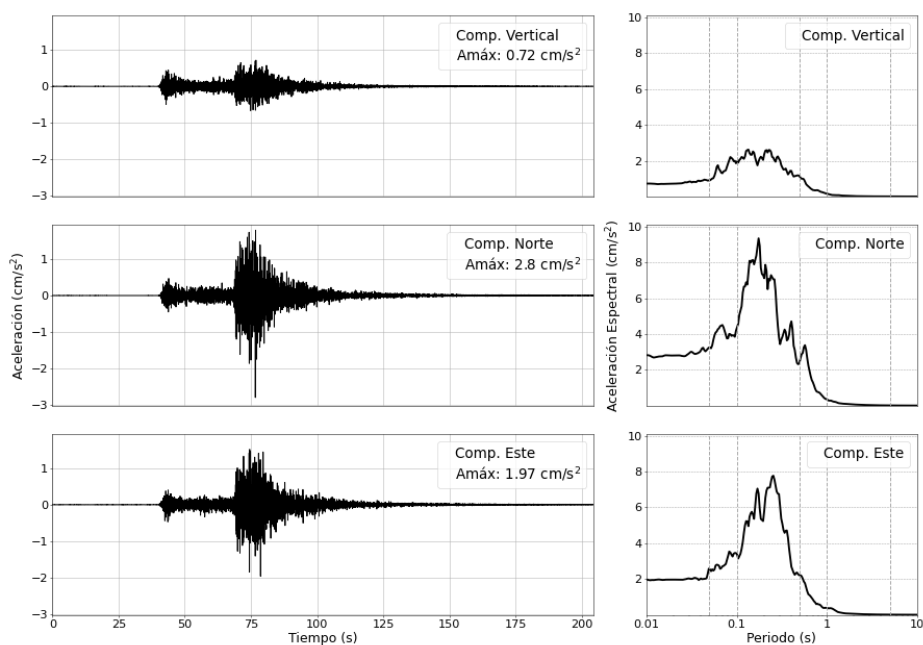
Figura 5: Registros de aceleración para el sismo del 23/08/2025 (M5.2) y sus correspondientes espectros de respuestas con amortiguamiento al 5 %
