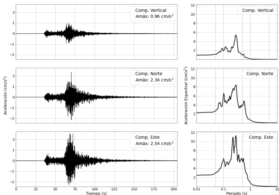
Figura 4: Registros de aceleración para el sismo del 23/08/2025 (M5.2) y sus correspondientes espectros de respuestas con amortiguamiento al 5 %
