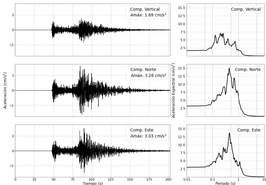
Figura 4: Registros de aceleración para el sismo del 25/09/2025 (M5.2) y sus correspondientes espectros de respuestas con amortiguamiento al 5 %
