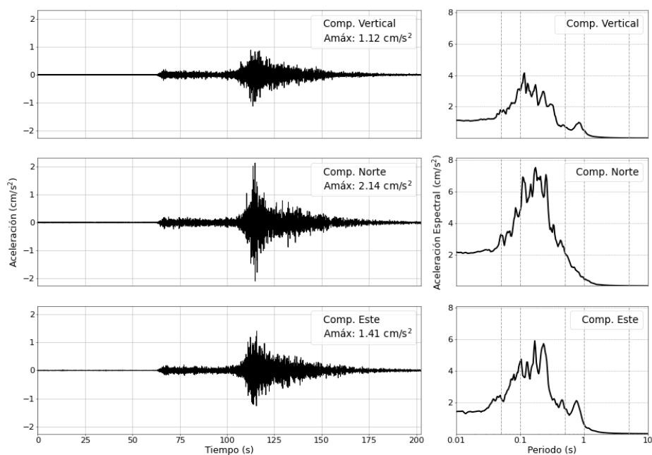
Figura 6: Registro de aceleración para el sismo del 25/09/2025 (M5.2) y sus correspondientes espectros de respuestas con amortiguamiento al 5 %
