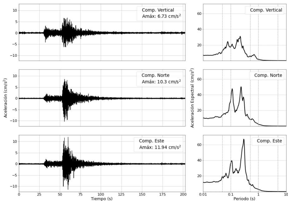
Figura 3: Registros de aceleración para el sismo del 25/09/2025 (M5.2) y sus correspondientes espectros de respuestas con amortiguamiento al 5 %
