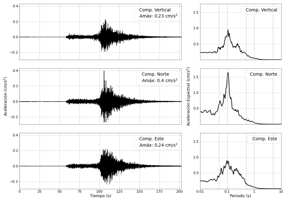
Figura 5: Registros de aceleración para el sismo del 25/09/2025 ( M_{5.2} ) y sus correspondientes espectros de respuestas con amortiguamiento al 5 %
