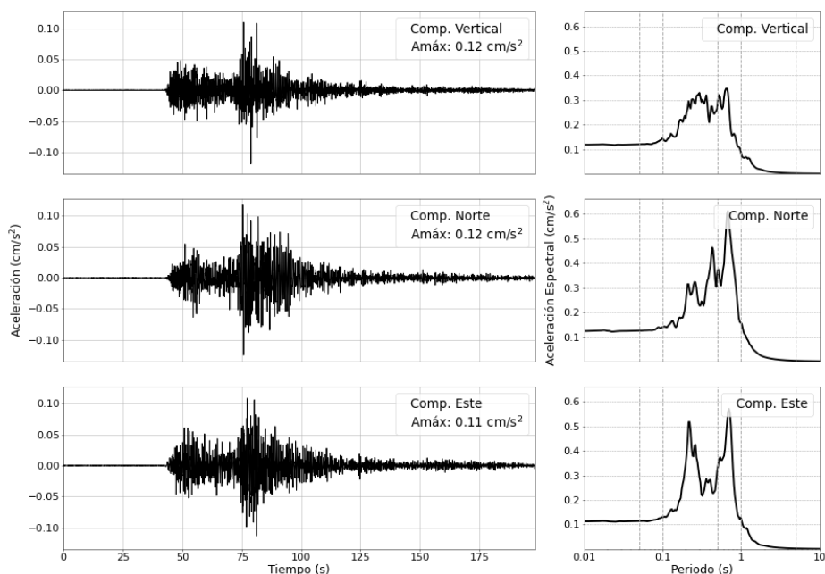
Figura 5: Registros de aceleración para el sismo del 12/09/2025 ( M_{4.9} ) y sus correspondientes espectros de respuestas con amortiguamiento al 5 %
