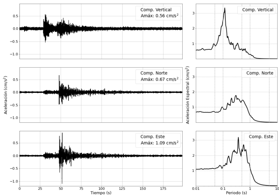
Figura 3: Registros de aceleración para el sismo del 12/09/2025 (M4.9) y sus correspondientes espectros de respuestas con amortiguamiento al 5 %
