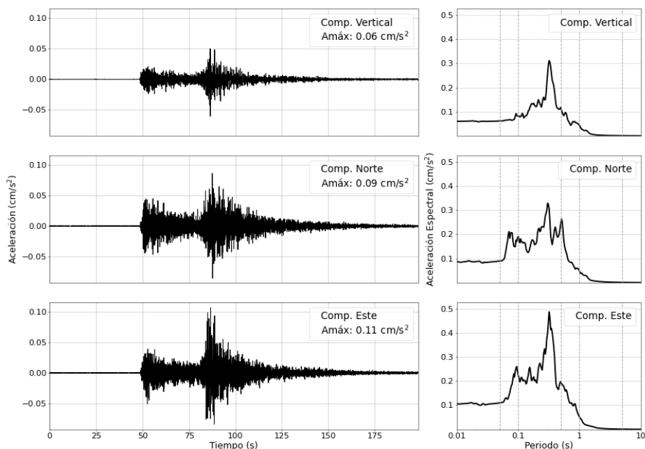
Figura 6: Registros de aceleración para el sismo del 12/09/2025 (M4.9) y sus correspondientes espectros de respuestas con amortiguamiento al 5 %
