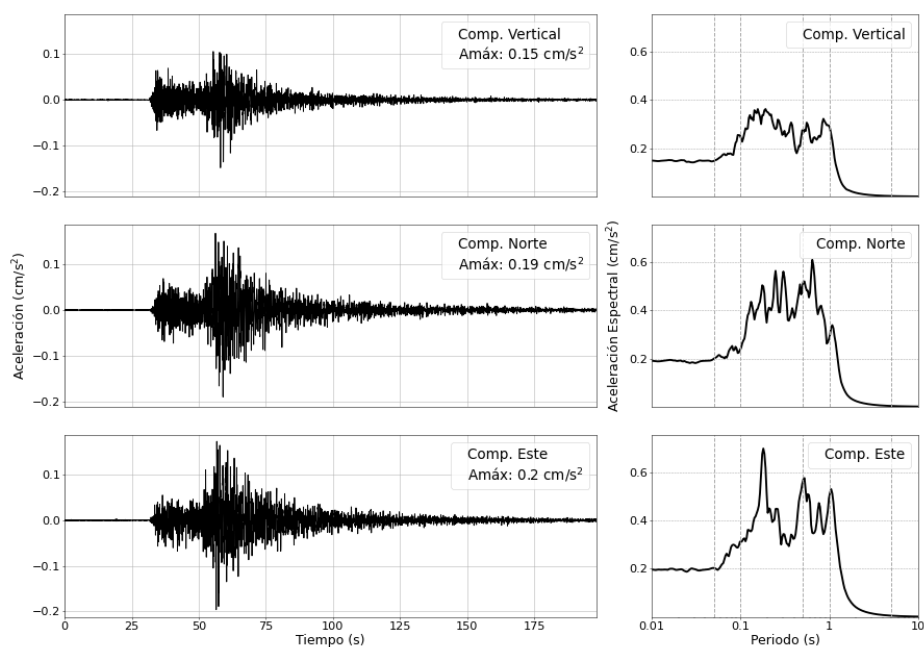
Figura 4: Registros de aceleración para el sismo del 12/09/2025 (M4.9) y sus correspondientes espectros de respuestas con amortiguamiento al 5 %
