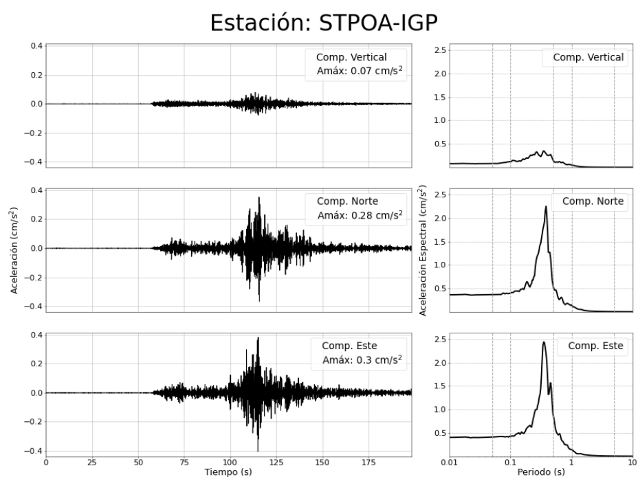
Figura 7: Registro de aceleracion para el sismo del 12/09/2025 (M4.9) y sus correspondientes espectros de respuestas con amortiguamiento al 5 %
