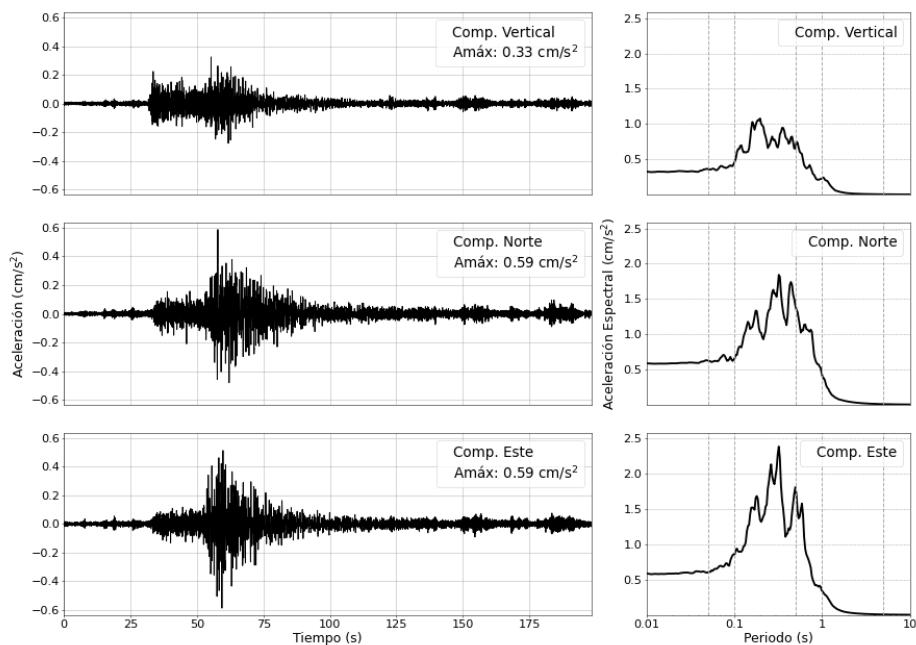
Figura 3: Registros de aceleración para el sismo del 20/03/2026 ( M4.9 ) y sus correspondientes espectros de respuestas con amortiguamiento al 5 %
