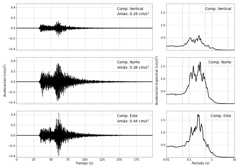
Figura 4: Registros de aceleración para el sismo del 20/03/2026 ( M4.9 ) y sus correspondientes espectros de respuestas con amortiguamiento al 5 %
