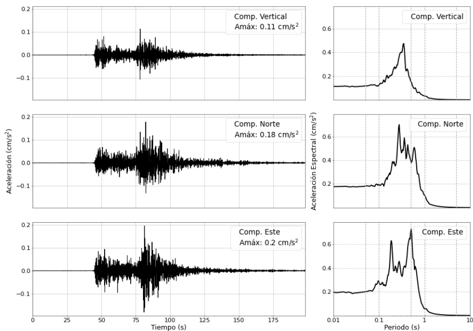
Figura 6: Registros de aceleración para el sismo del 20/03/2026 (M4.9) y sus correspondientes espectros de respuestas con amortiguamiento al 5 %
