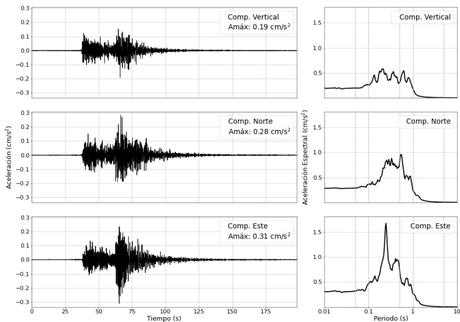
Figura 5: Registros de aceleración para el sismo del 20/03/2026 ( M4.9 ) y sus correspondientes espectros de respuestas con amortiguamiento al 5 %
