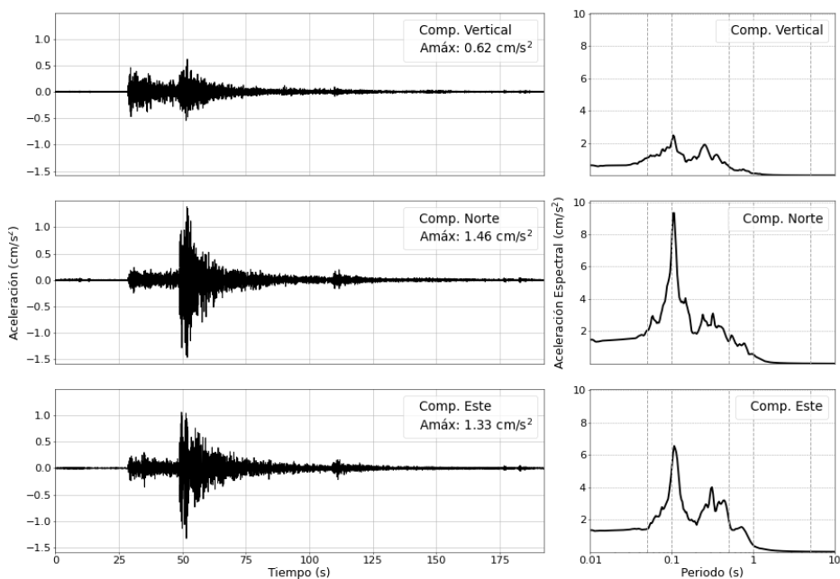
Figura 5: Registros de aceleración para el sismo del 07/03/2026 (M4.9) y sus correspondientes espectros de respuestas con amortiguamiento al 5 %
