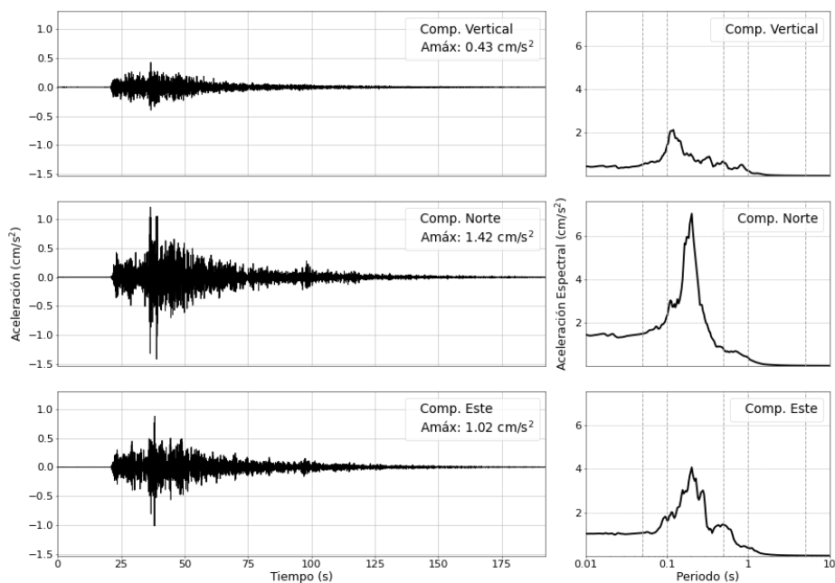
Figura 3: Registros de aceleración para el sismo del 07/03/2026 (M4.9) y sus correspondientes espectros de respuestas con amortiguamiento al 5 %
