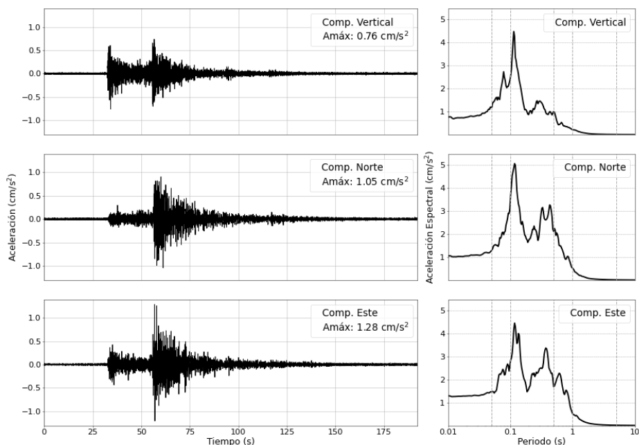
Figura 7: Registros de aceleración para el sismo del 07/03/2026 (M4.9) y sus correspondientes espectros de respuestas con amortiguamiento al 5 %
