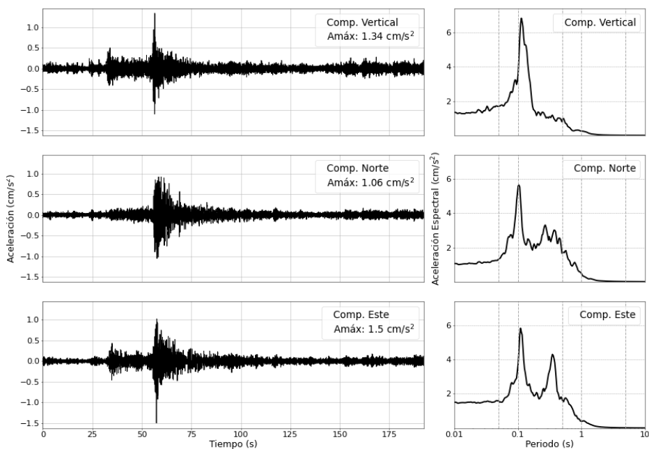
Figura 6: Registros de aceleración para el sismo del 07/03/2026 (M4.9) y sus correspondientes espectros de respuestas con amortiguamiento al 5 %
