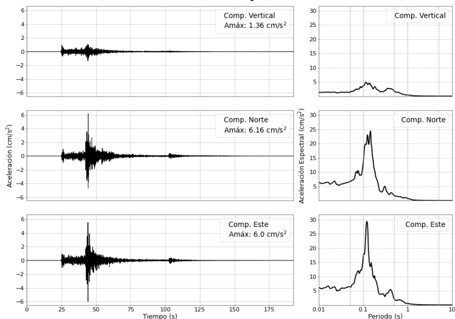
Figura 4: Registros de aceleración para el sismo del 07/03/2026 (M4.9) y sus correspondientes espectros de respuestas con amortiguamiento al 5 %
