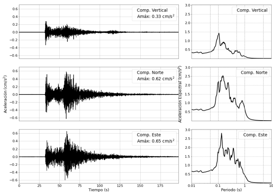
Figura 5: Registros de aceleración para el sismo del 11/10/2025 ( M_{4.9} ) y sus correspondientes espectros de respuestas con amortiguamiento al 5 %
