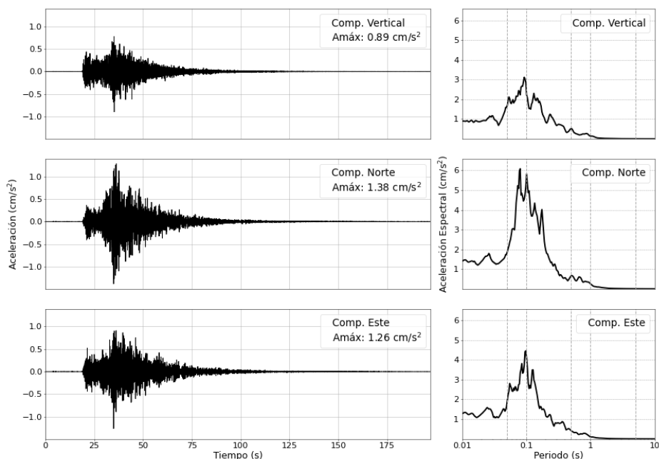
Figura 4: Registros de aceleración para el sismo del 11/10/2025 (M4.9) y sus correspondientes espectros de respuestas con amortiguamiento al 5 %
