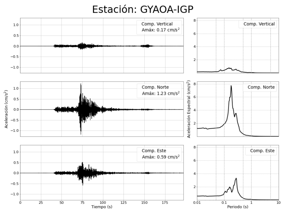
Figura 6: Registro de aceleración para el sismo del 11/10/2025 (M4.9) y sus correspondientes espectros de respuestas con amortiguamiento al 5 %
