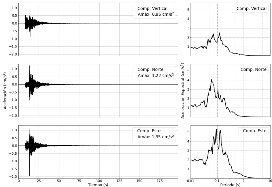
Figura 3: Registros de aceleración para el sismo del 11/10/2025 (M4.9) y sus correspondientes espectros de respuestas con amortiguamiento al 5 %
