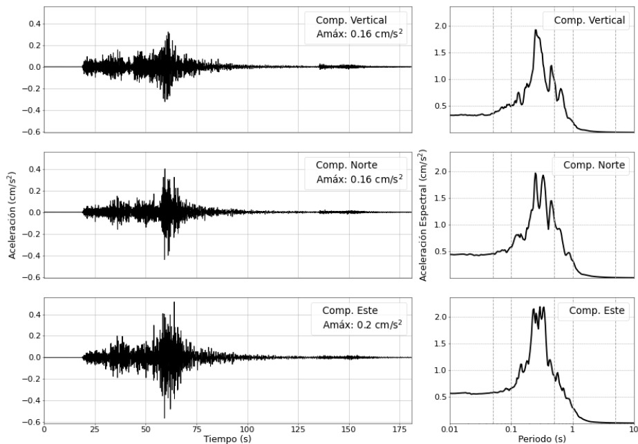
Figura 3: Registros de aceleración para el sismo del 23/03/2026 ( M_{4.8} ) y sus correspondientes espectros de respuestas con amortiguamiento al 5 %
