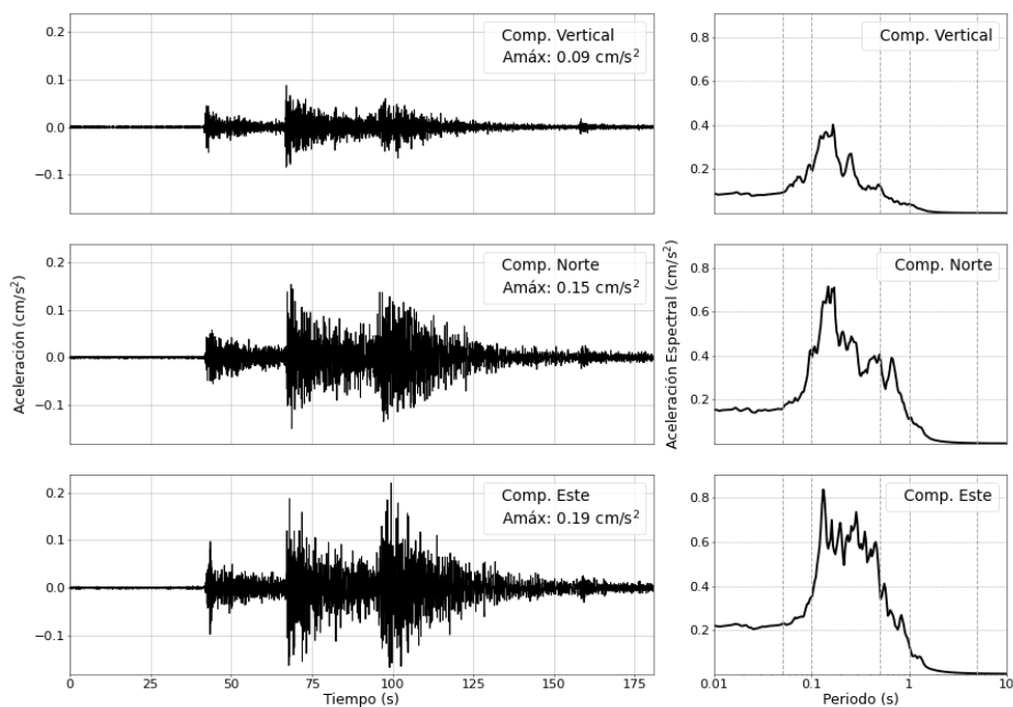
Figura 4: Registros de aceleración para el sismo del 23/03/2026 (M4.8) y sus correspondientes espectros de respuestas con amortiguamiento al 5 %
