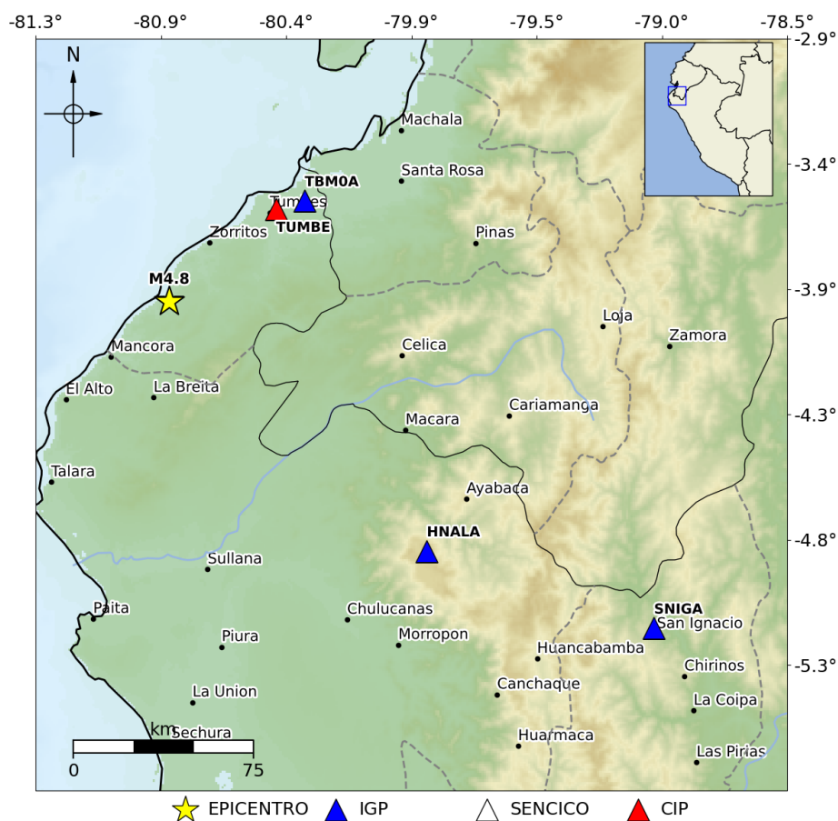
Figura 1: Epicentro del sismo ocurrido el 23/03/2026 y distribución de las estaciones acelerométricas consideradas en este reporte
