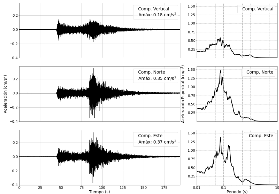
Figura 3: Registros de aceleración para el sismo del 13/01/2026 (M4.8) y sus correspondientes espectros de respuestas con amortiguamiento al 5 %
