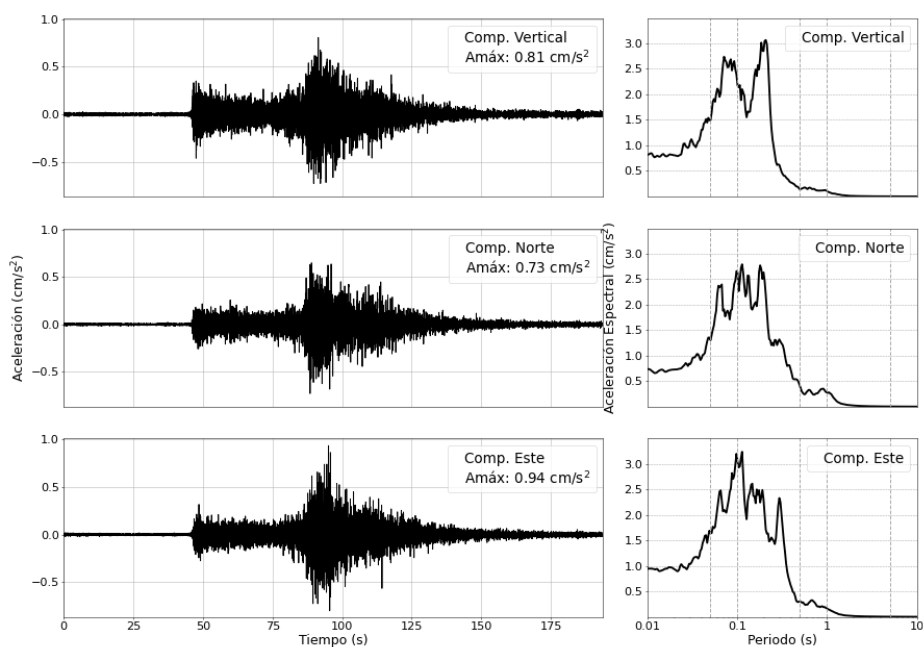
Figura 4: Registros de aceleracion para el sismo del 13/01/2026 (M4.8) y sus correspondientes espectros de respuestas con amortiguamiento al 5 %
