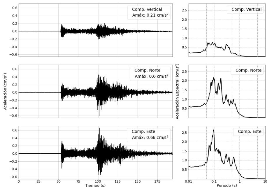
Figura 5: Registros de aceleración para el sismo del 13/01/2026 (M4.8) y sus correspondientes espectros de respuestas con amortiguamiento al 5 %
