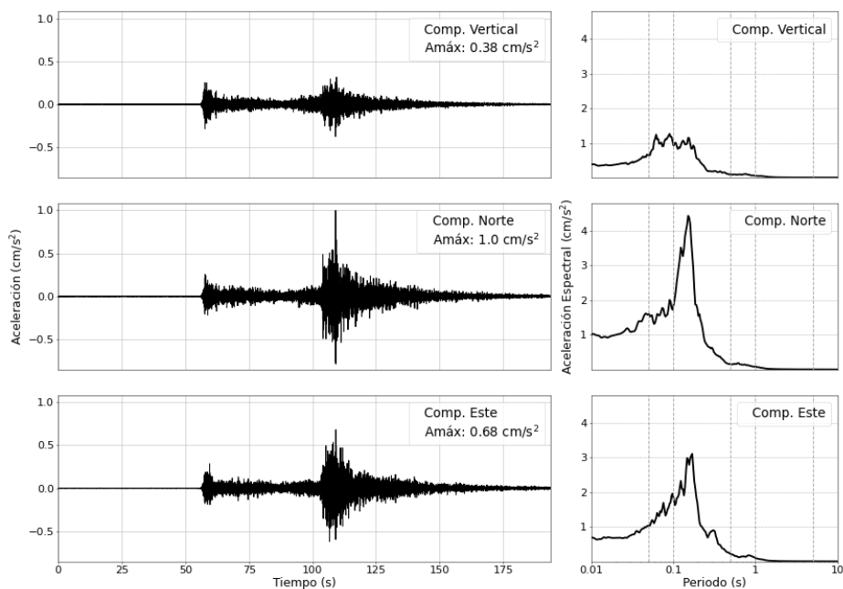
Figura 6: Registros de aceleración para el sismo del 13/01/2026 (M4.8) y sus correspondientes espectros de respuestas con amortiguamiento al 5 %
