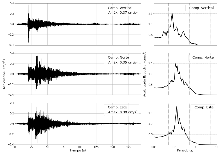
Figura 3: Registros de aceleración para el sismo del 07/09/2025 (M4.7) y sus correspondientes espectros de respuestas con amortiguamiento al 5 %
