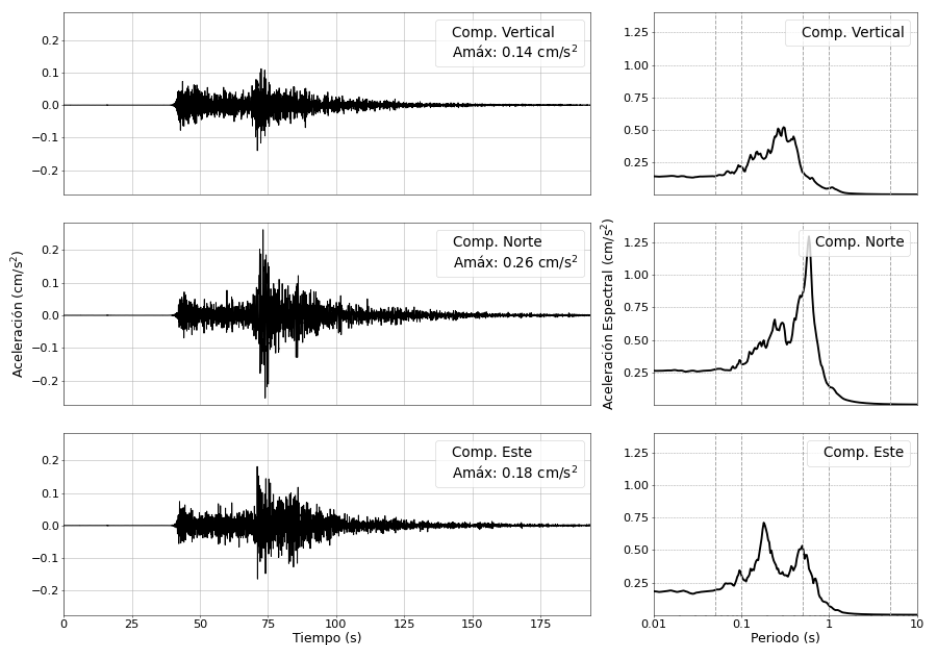
Figura 7: Registros de aceleracion para el sismo del 07/09/2025 (M4.7) y sus correspondientes espectros de respuestas con amortiguamiento al 5 %
