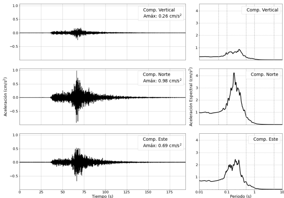
Figura 6: Registros de aceleración para el sismo del 07/09/2025 (M4.7) y sus correspondientes espectros de respuestas con amortiguamiento al 5 %
