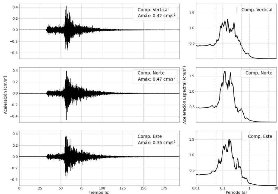
Figura 5: Registros de aceleración para el sismo del 07/09/2025 ( M4.7 ) y sus correspondientes espectros de respuestas con amortiguamiento al 5 %
