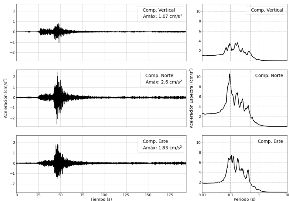
Figura 4: Registros de aceleracion para el sismo del 07/09/2025 (M4.7) y sus correspondientes espectros de respuestas con amortiguamiento al 5 %
