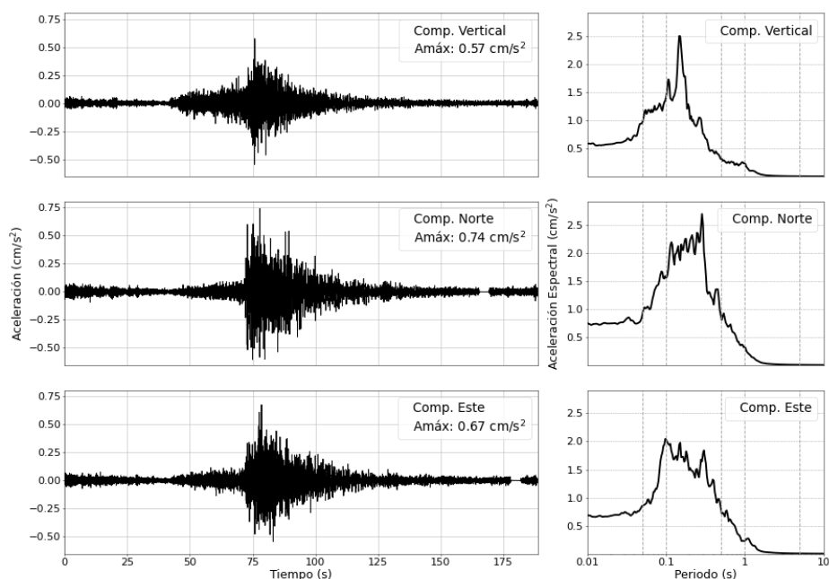
Figura 7: Registros de aceleracion para el sismo del 25/09/2025 (M4.6) y sus correspondientes espectros de respuestas con amortiguamiento al 5 %
