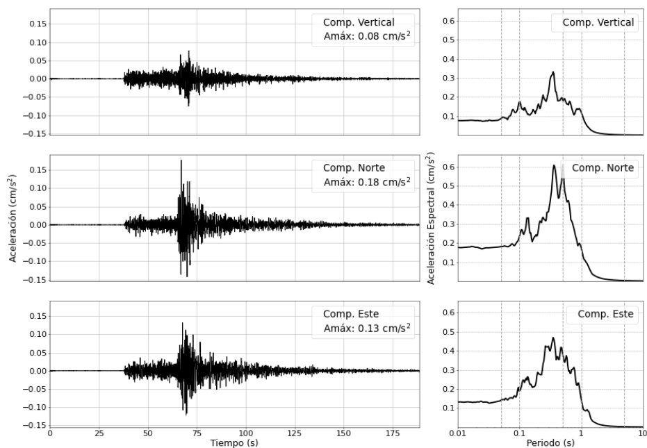
Figura 6: Registros de aceleración para el sismo del 25/09/2025 (M4.6) y sus correspondientes espectros de respuestas con amortiguamiento al 5 %
