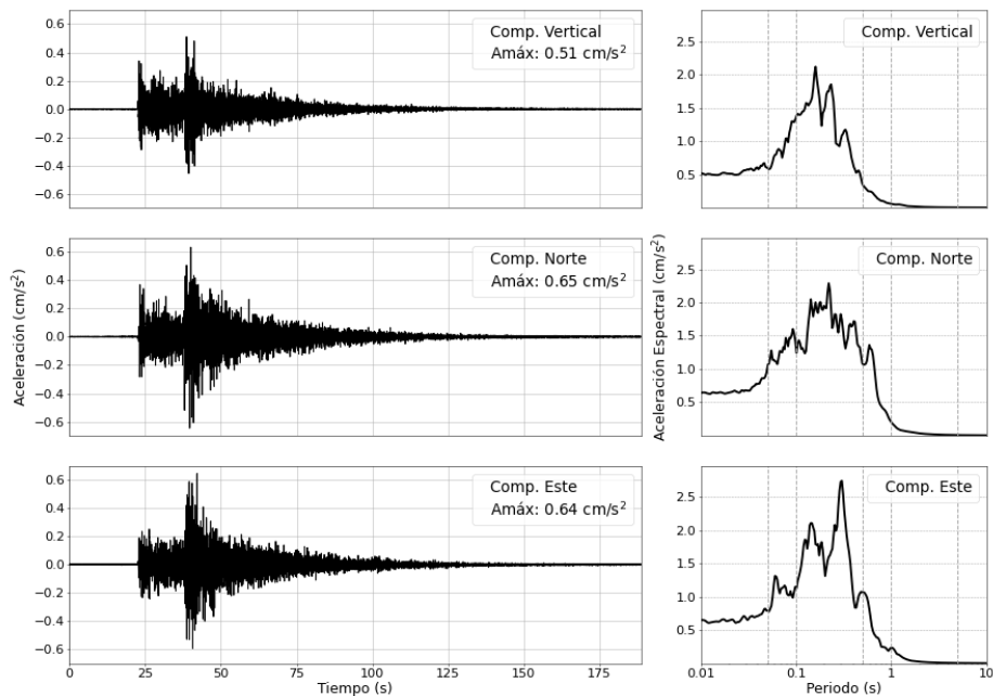
Figura 3: Registros de aceleración para el sismo del 25/09/2025 (M4.6) y sus correspondientes espectros de respuestas con amortiguamiento al 5 %
