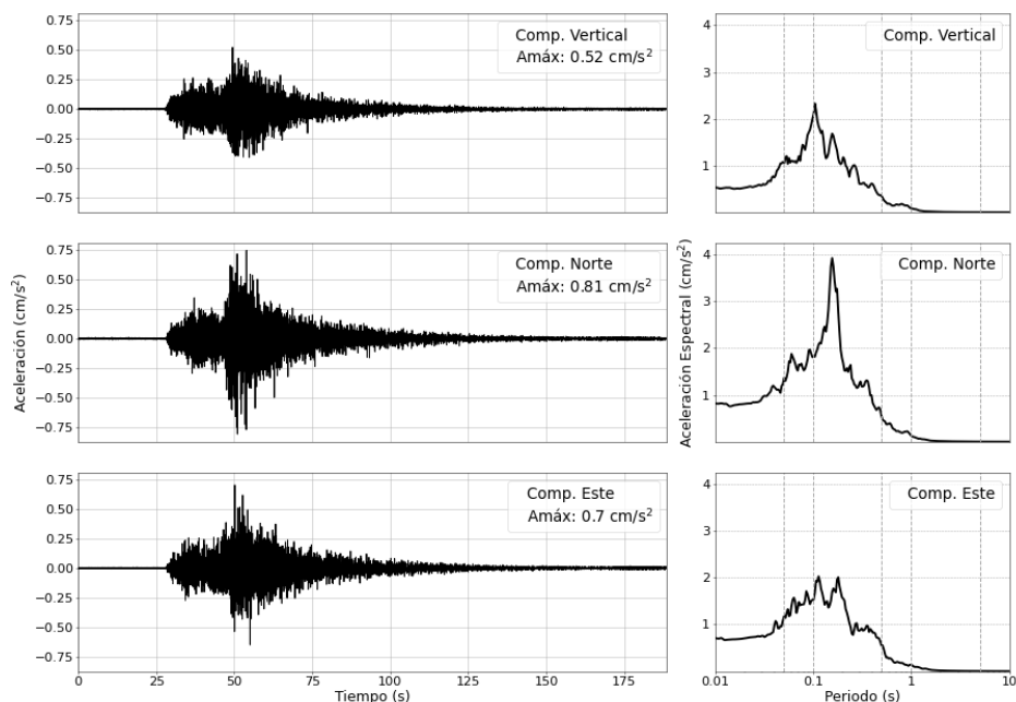
Figura 5: Registros de aceleración para el sismo del 25/09/2025 (M4.6) y sus correspondientes espectros de respuestas con amortiguamiento al 5 %
