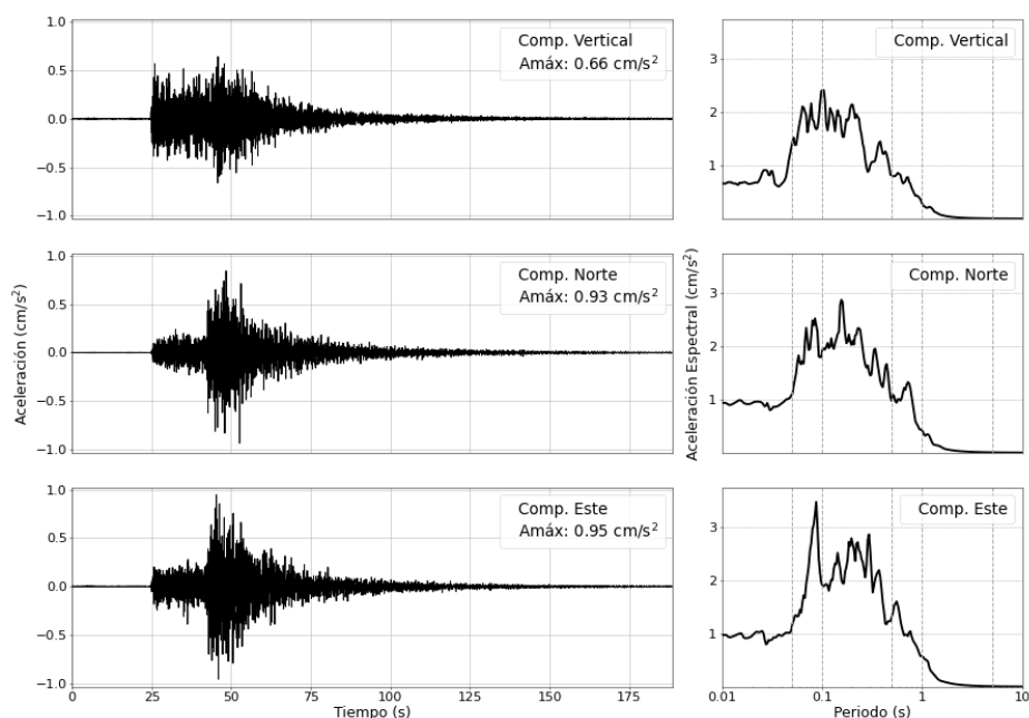
Figura 4: Registros de aceleración para el sismo del 25/09/2025 (M4.6) y sus correspondientes espectros de respuestas con amortiguamiento al 5 %
