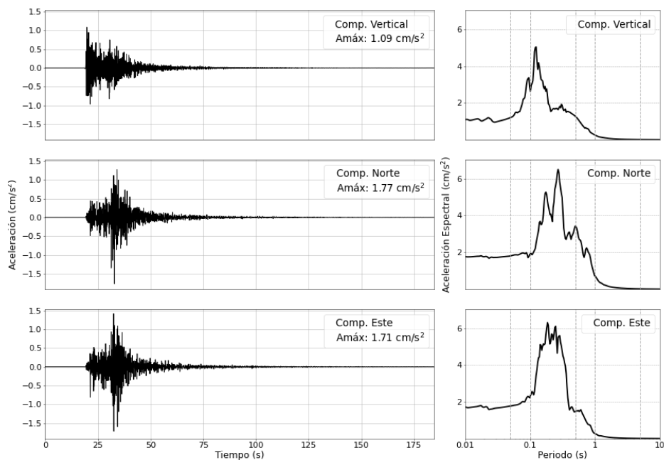
Figura 3: Registros de aceleración para el sismo del 26/08/2025 ( M_{4.6} ) y sus correspondientes espectros de respuestas con amortiguamiento al 5 %
