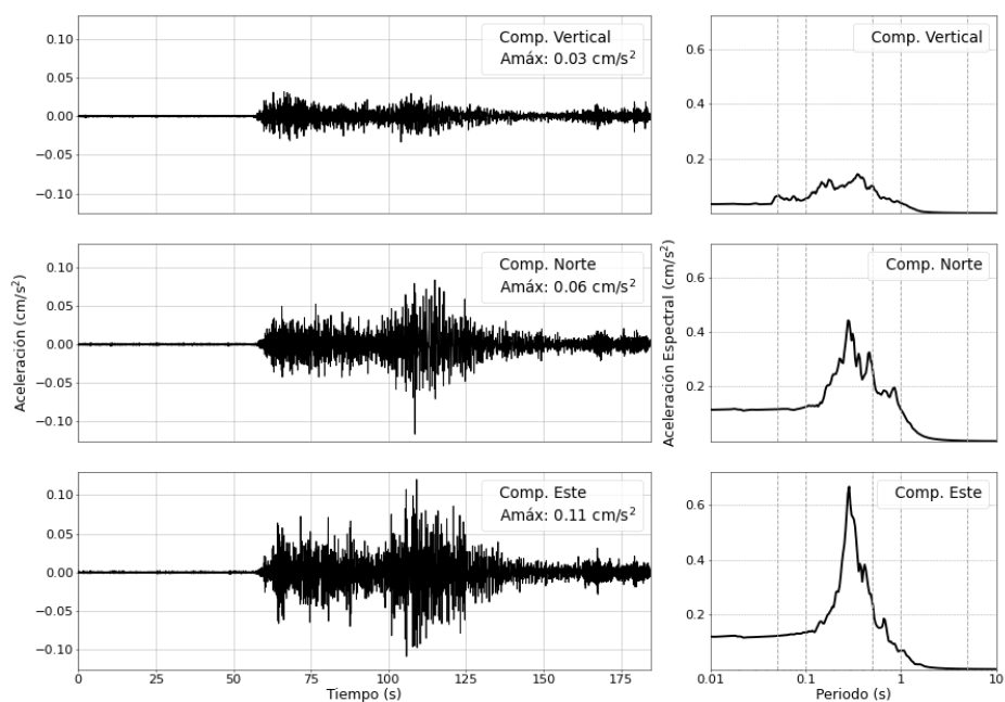
Figura 6: Registro de aceleracion para el sismo del 26/08/2025 (M4.6) y sus correspondientes espectros de respuestas con amortiguamiento al 5 %
