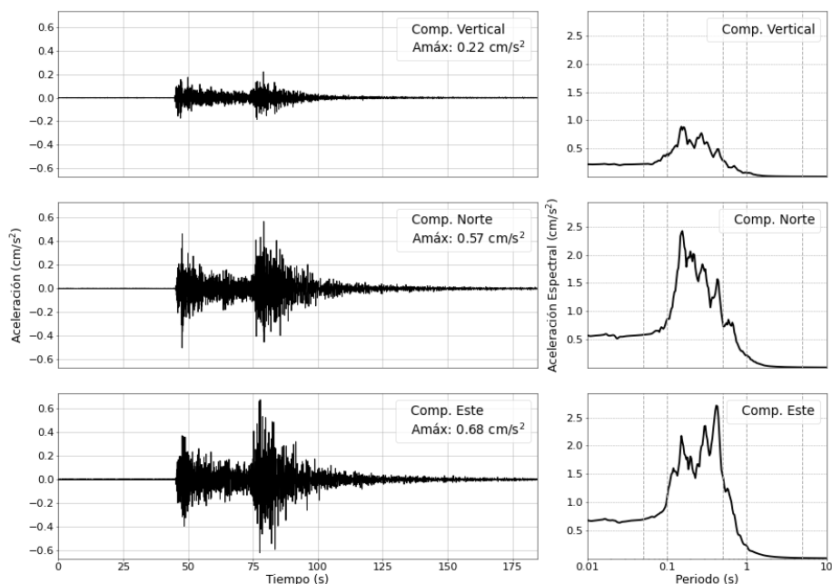
Figura 5: Registros de aceleración para el sismo del 26/08/2025 (M4.6) y sus correspondientes espectros de respuestas con amortiguamiento al 5 %
