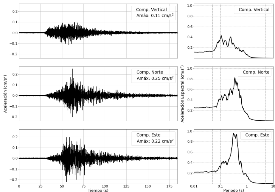
Figura 4: Registros de aceleración para el sismo del 26/08/2025 (M4.6) y sus correspondientes espectros de respuestas con amortiguamiento al 5 %
