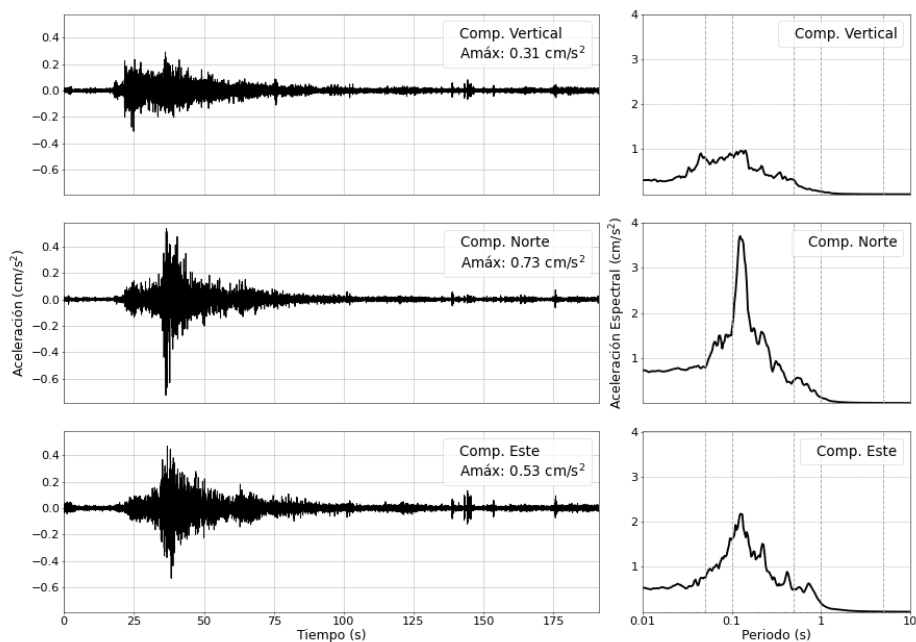
Figura 3: Registros de aceleración para el sismo del 24/09/2025 ( M_{4.6} ) y sus correspondientes espectros de respuestas con amortiguamiento al 5 %
