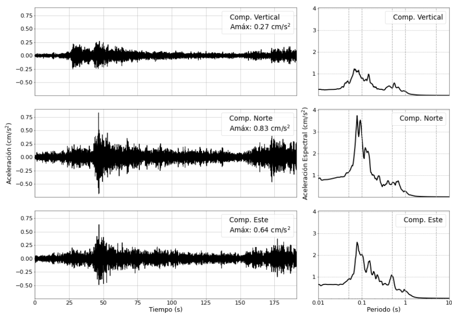
Figura 4: Registros de aceleración para el sismo del 24/09/2025 (M4.6) y sus correspondientes espectros de respuestas con amortiguamiento al 5 %
