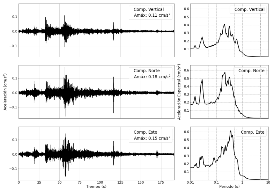
Figura 5: Registros de aceleración para el sismo del 24/09/2025 (M4.6) y sus correspondientes espectros de respuestas con amortiguamiento al 5 %
