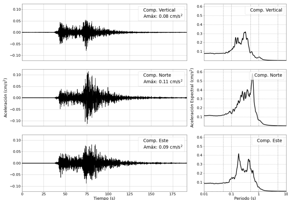
Figura 6: Registros de aceleracion para el sismo del 24/09/2025 (M4.6) y sus correspondientes espectros de respuestas con amortiguamiento al 5 %
