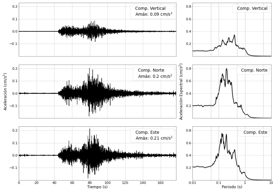
Figura 3: Registros de aceleración para el sismo del 09/06/2026 (M4.5) y sus correspondientes espectros de respuestas con amortiguamiento al 5 %
