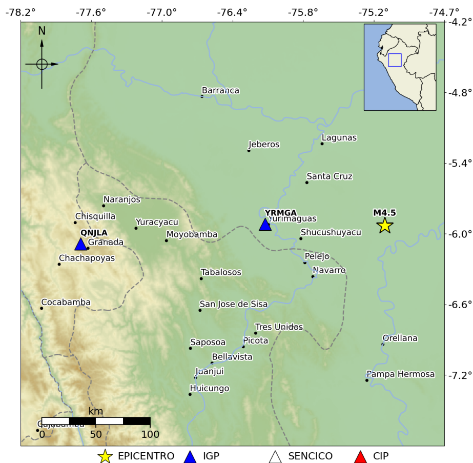
Figura 1: Epicentro del sismo ocurrido el 09/06/2026 y distribución de las estaciones acelerométricas consideradas en este reporte
