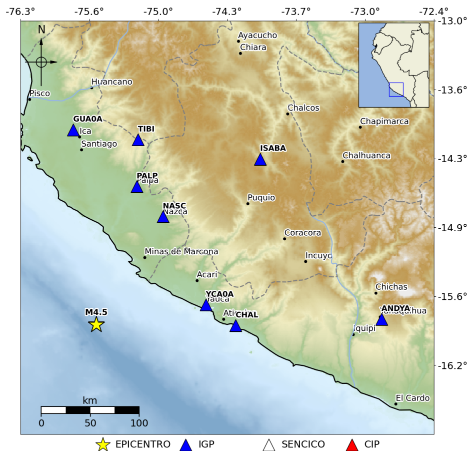
Figura 1: Epicentro del sismo ocurrido el 05/06/2026 y distribución de las estaciones acelerométricas consideradas en este reporte
