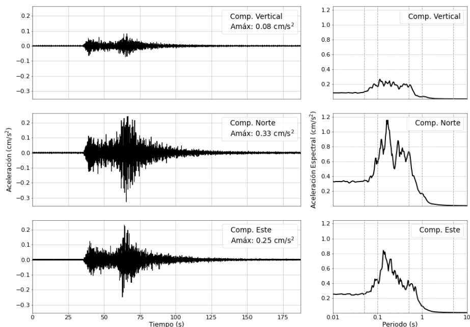
Figura 5: Registros de aceleración para el sismo del 05/06/2026 ( M4.5 ) y sus correspondientes espectros de respuestas con amortiguamiento al 5 %
