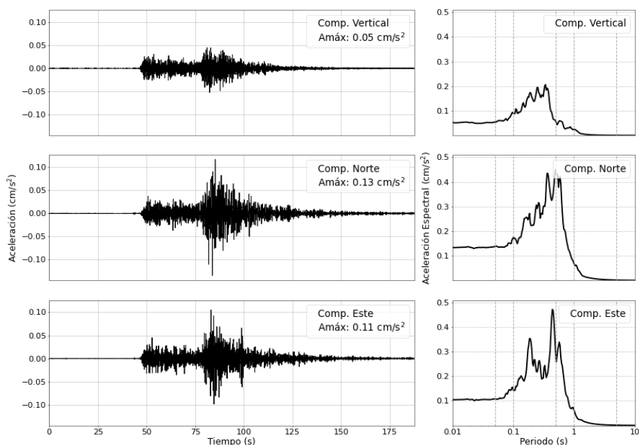
Figura 6: Registros de aceleración para el sismo del 05/06/2026 (M4.5) y sus correspondientes espectros de respuestas con amortiguamiento al 5 %
