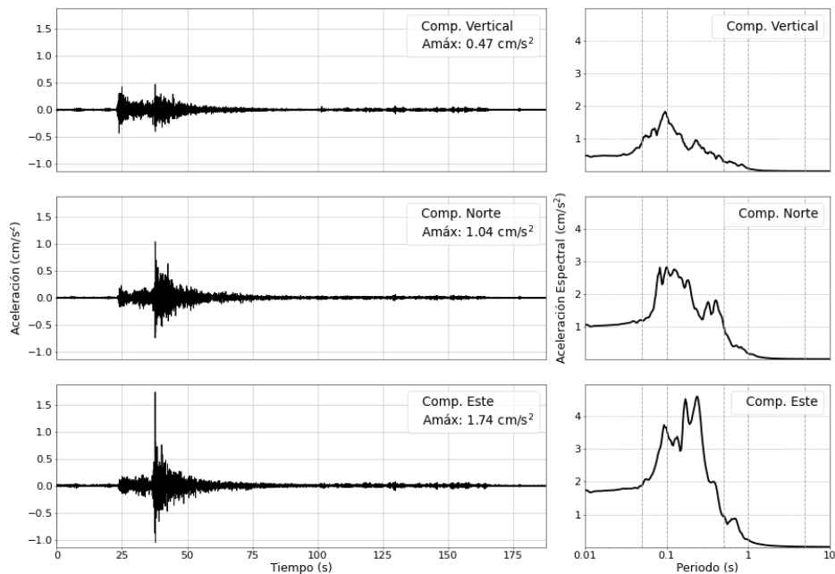
Figura 3: Registros de aceleración para el sismo del 05/06/2026 ( M_{4.5} ) y sus correspondientes espectros de respuestas con amortiguamiento al 5 %
