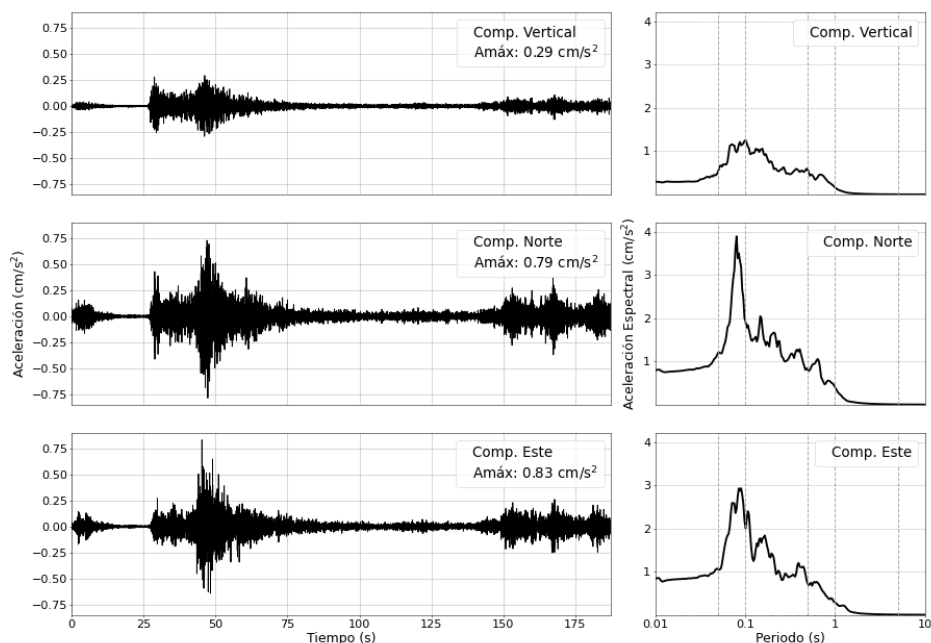
Figura 4: Registros de aceleración para el sismo del 05/06/2026 (M4.5) y sus correspondientes espectros de respuestas con amortiguamiento al 5 %
