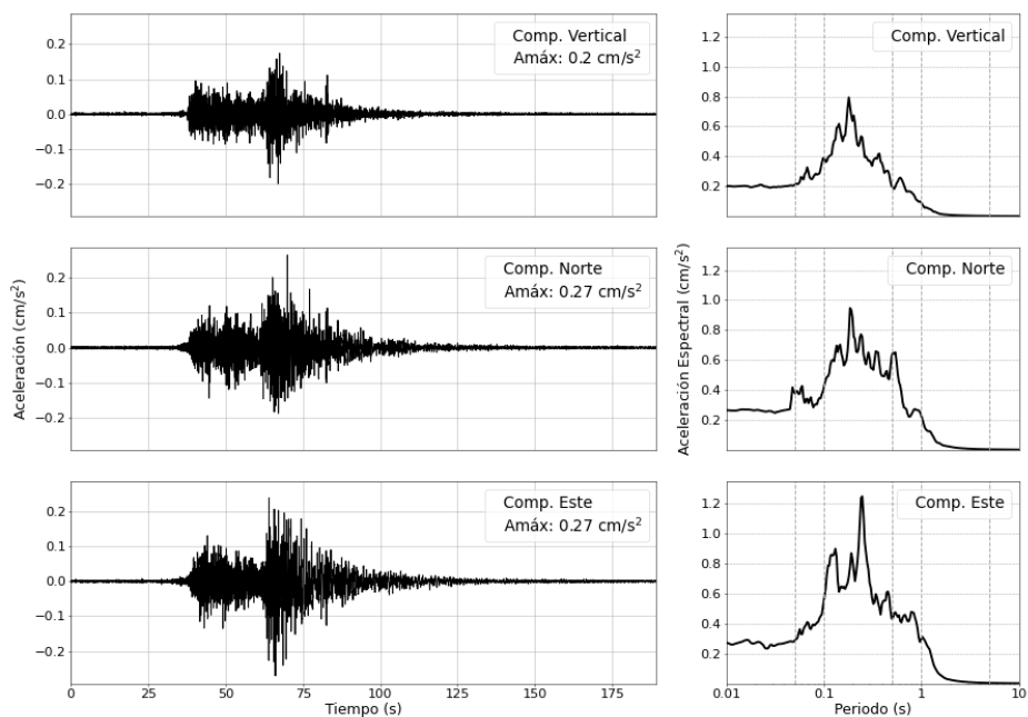
Figura 5: Registros de aceleracion para el sismo del 23/09/2025 (M4.5) y sus correspondientes espectros de respuestas con amortiguamiento al 5 %
