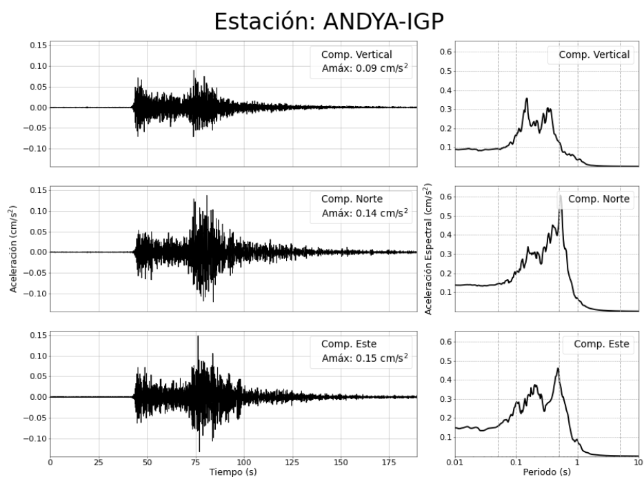
Figura 6: Registro de aceleración para el sismo del 23/09/2025 (M4.5) y sus correspondientes espectros de respuestas con amortiguamiento al 5 %
