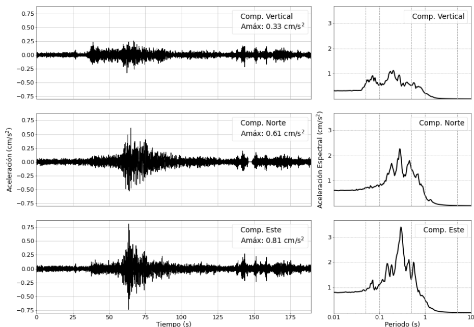
Figura 4: Registros de aceleración para el sismo del 23/09/2025 ( M4.5 ) y sus correspondientes espectros de respuestas con amortiguamiento al 5 %
