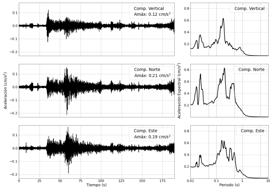
Figura 3: Registros de aceleración para el sismo del 23/09/2025 (M4.5) y sus correspondientes espectros de respuestas con amortiguamiento al 5 %
