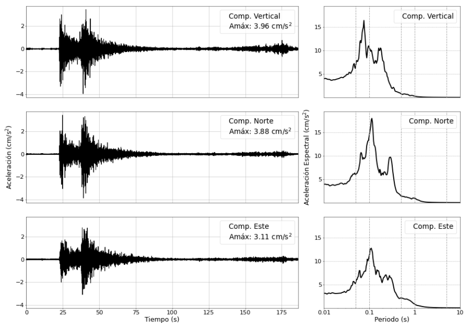
Figura 4: Registros de aceleración para el sismo del 04/04/2026 (M4.5) y sus correspondientes espectros de respuestas con amortiguamiento al 5 %
