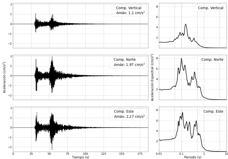
Figura 5: Registros de aceleración para el sismo del 04/04/2026 (M4.5) y sus correspondientes espectros de respuestas con amortiguamiento al 5 %
