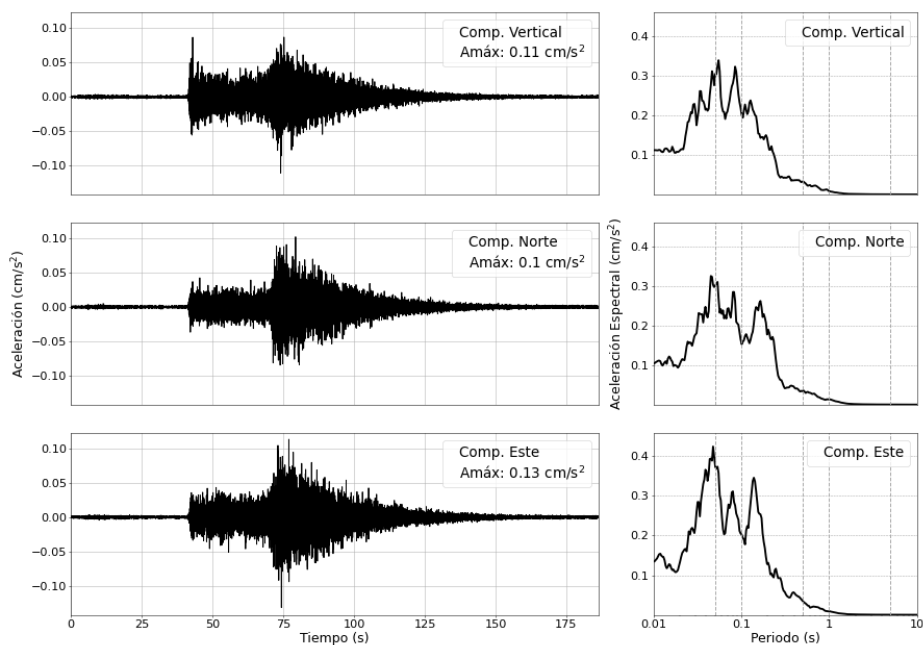
Figura 7: Registros de aceleracion para el sismo del 04/04/2026 (M4.5) y sus correspondientes espectros de respuestas con amortiguamiento al 5 %
