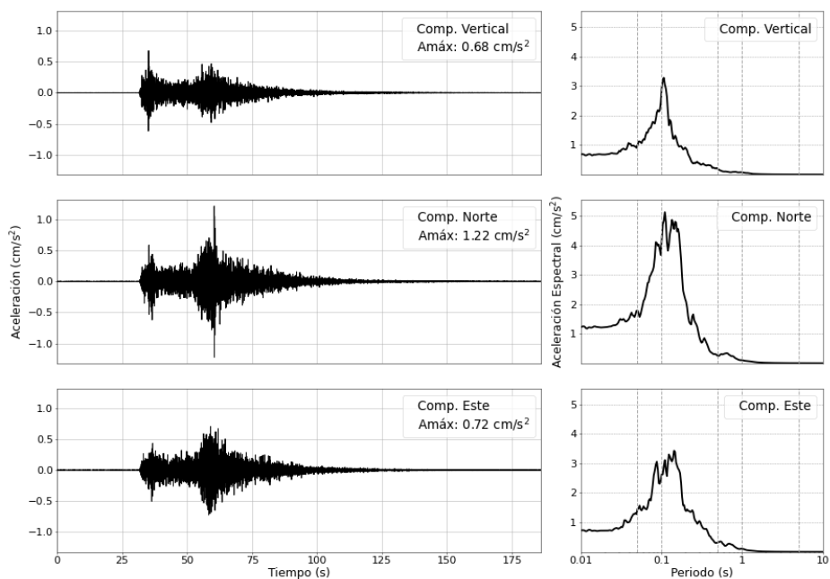
Figura 6: Registros de aceleración para el sismo del 04/04/2026 ( M_{4.5} ) y sus correspondientes espectros de respuestas con amortiguamiento al 5 %
